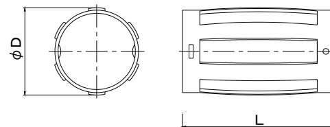
φ 17.8, φ 21.8用センタライザー
