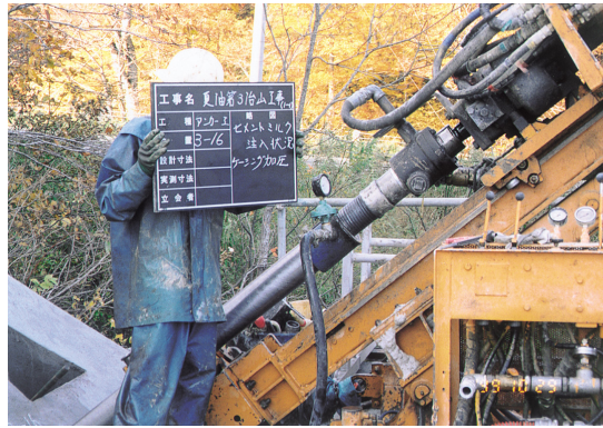
図 5.9.3 ケーシングヘッドによるケーシング加圧注入
