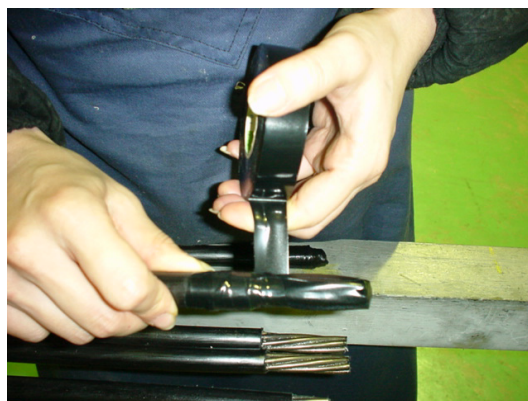
図 5.6.3 アンボンド PC 鋼より線の端部処理 （緊張端側）
