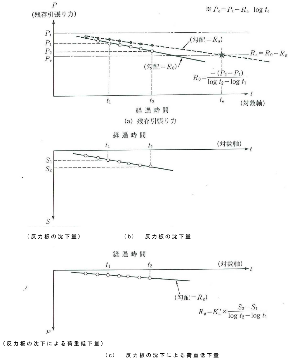
図 7.3.5 長期試験結果の一例
