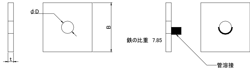
図 3.4.3 支圧板の形状
