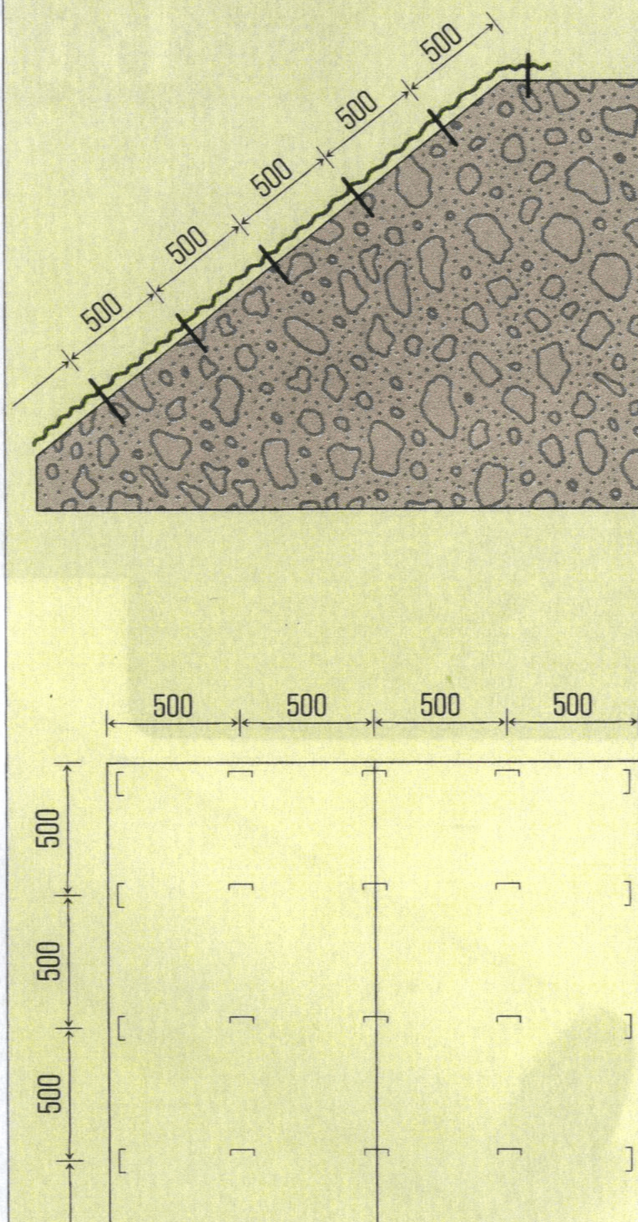
■施工例(アンカー打込位置図)
